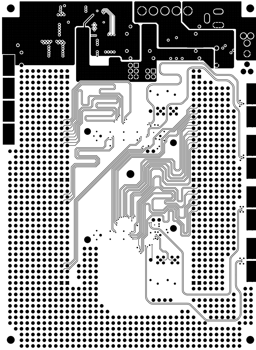
BOTTOM LAYER
