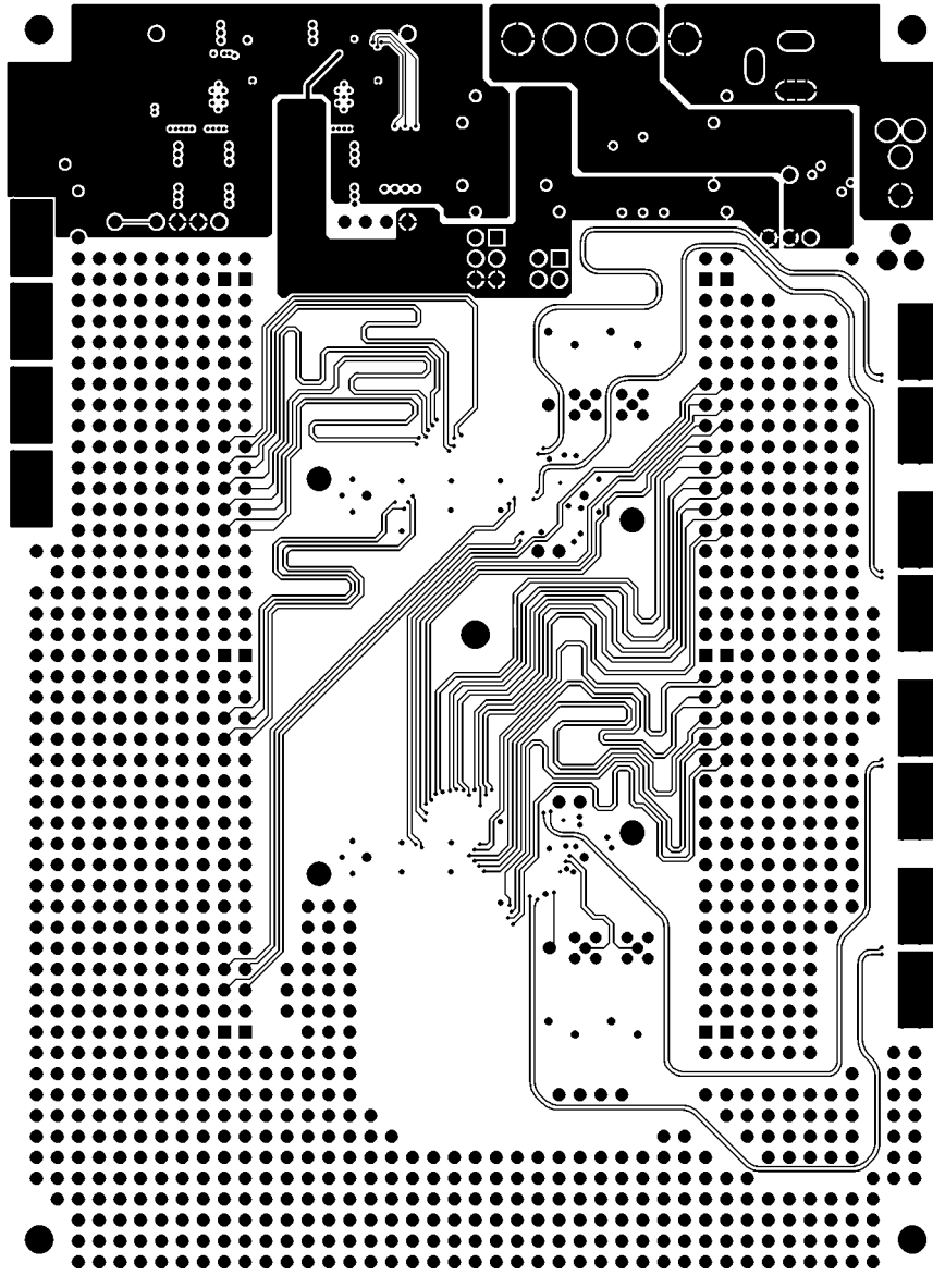
BOTTOM LAYER
