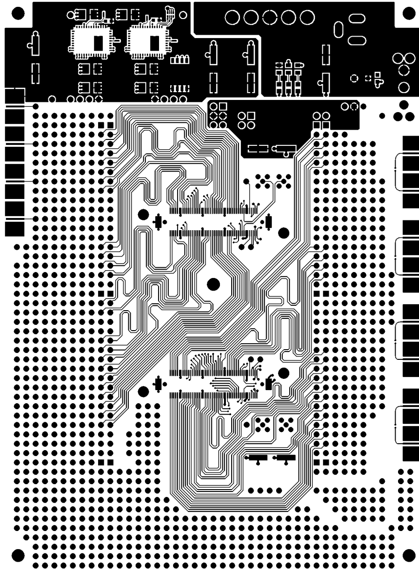
TOP LAYER
