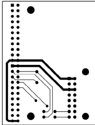
BOTTOM LAYER
