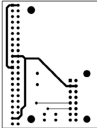
TOP LAYER
