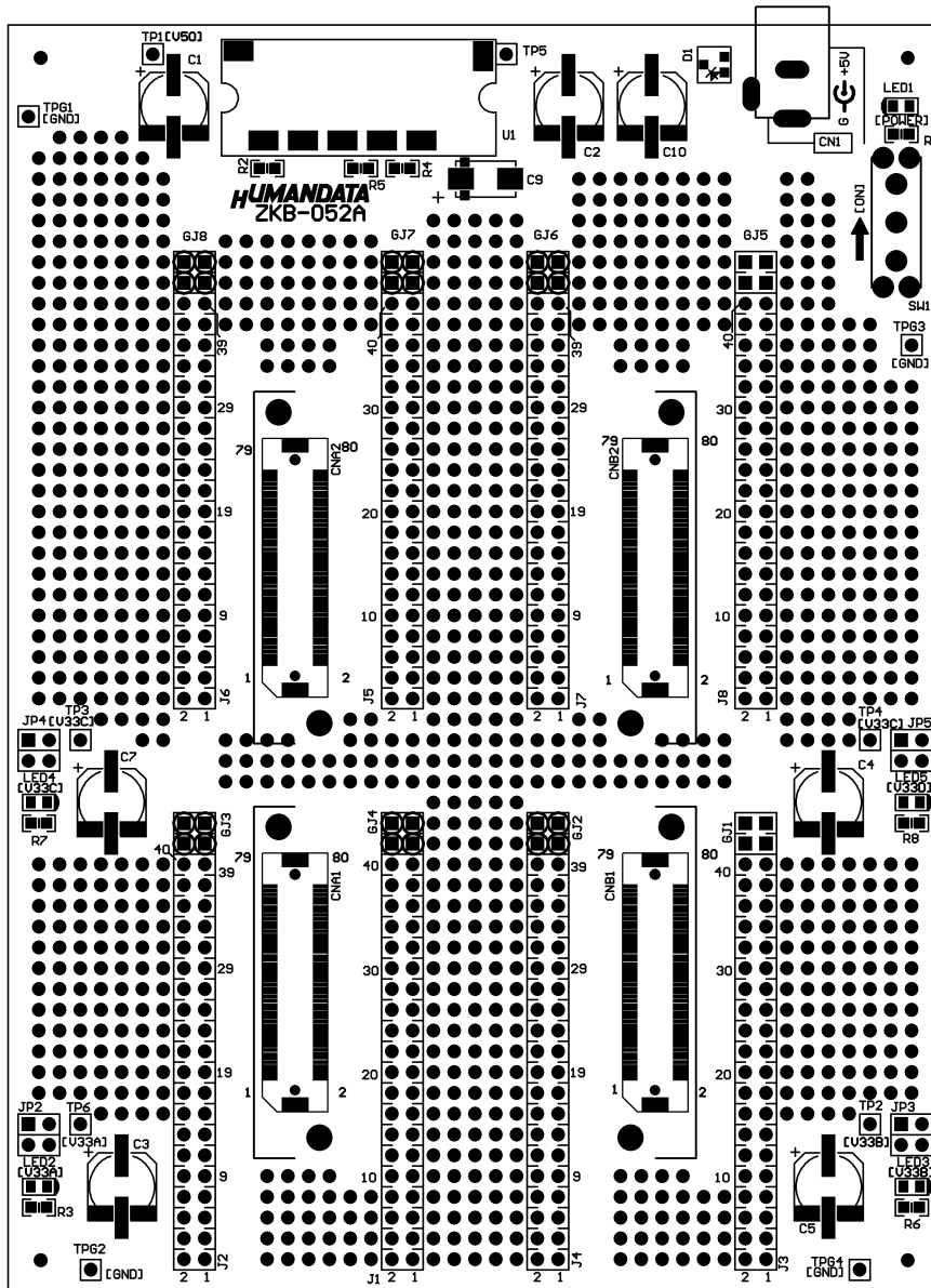
部品面
