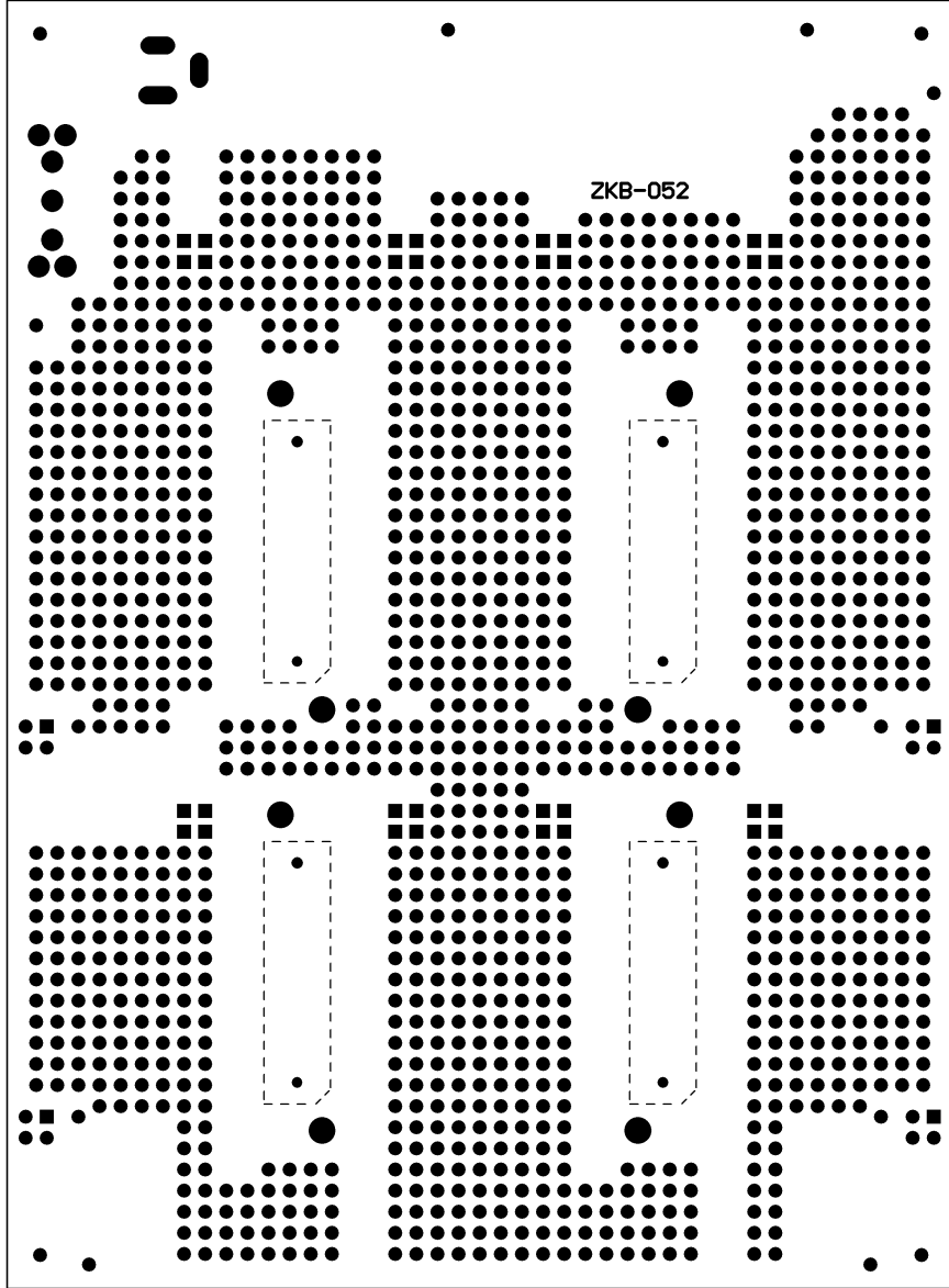
はんだ面
