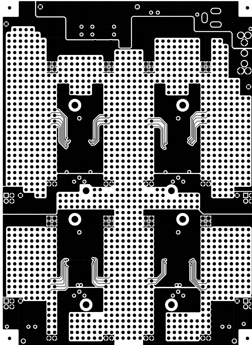
BOTTOM LAYER
