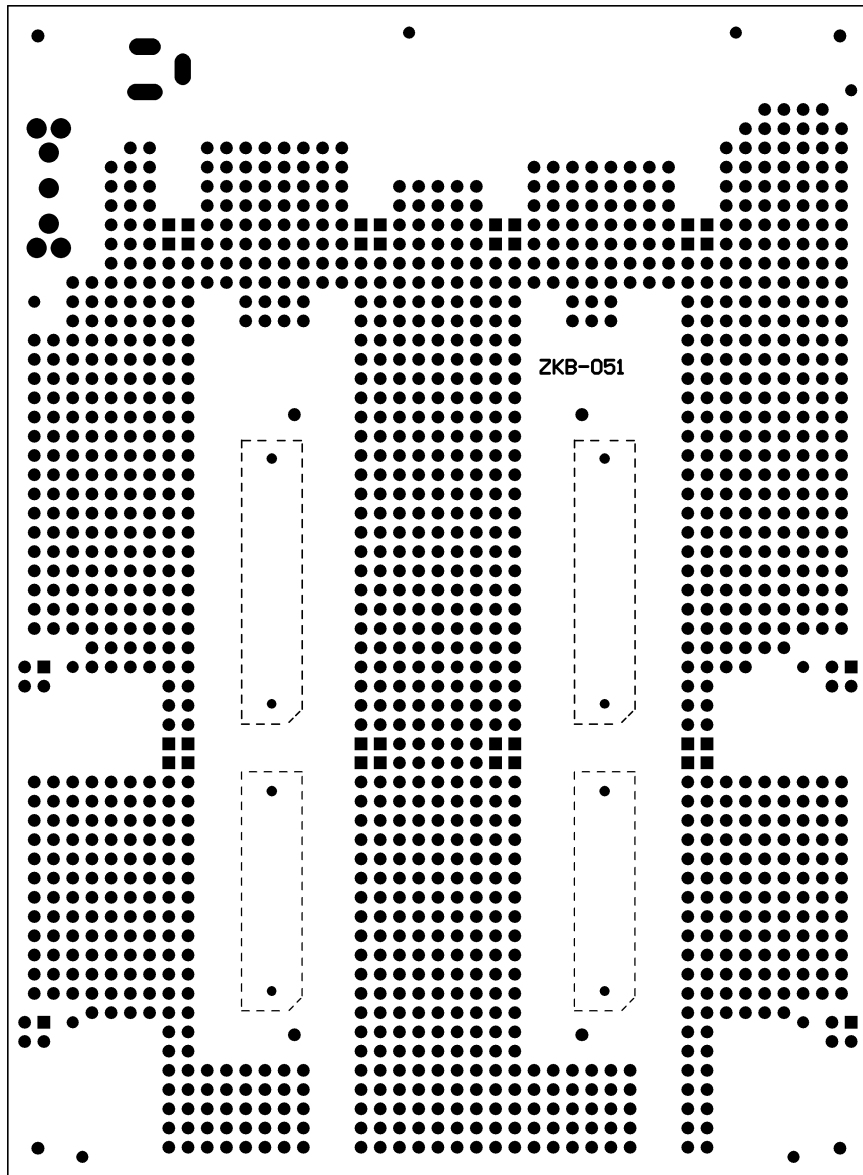
はんだ面
