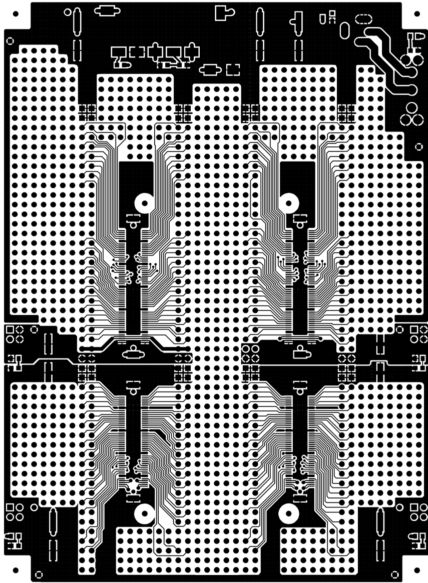
TOP LAYER
