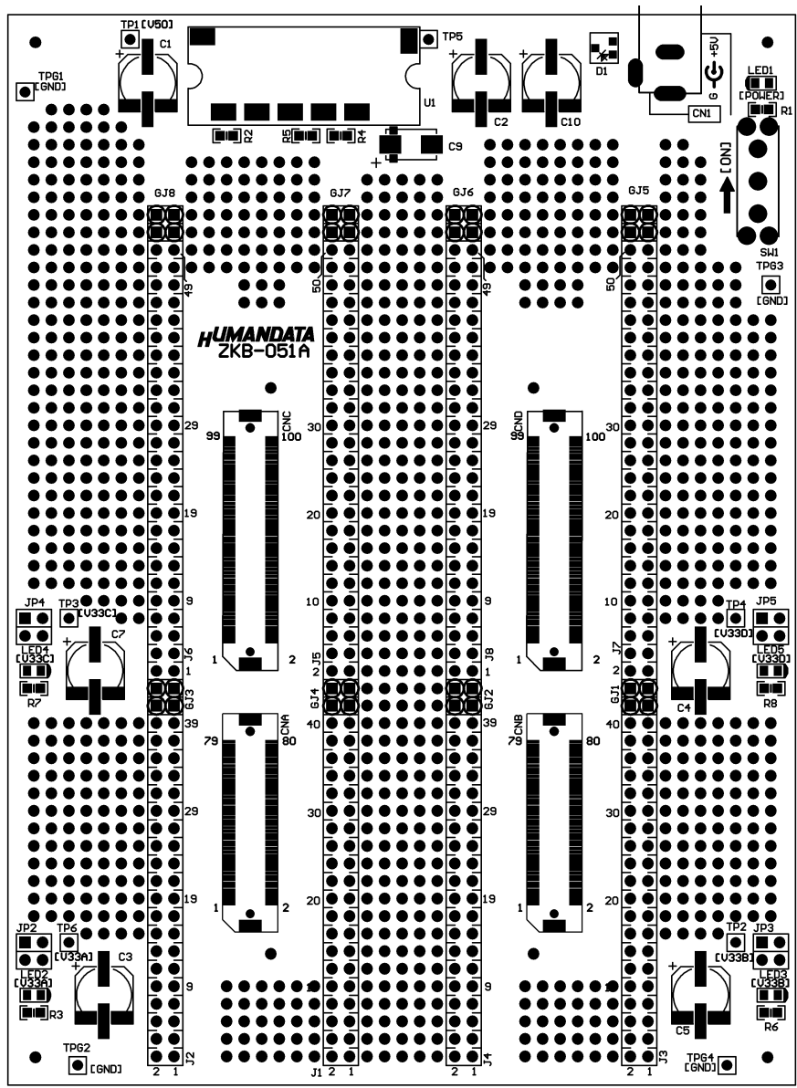
部品面
