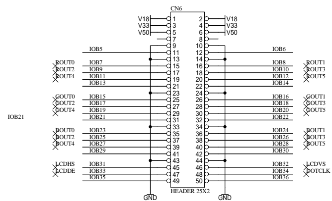
LCD I/F
