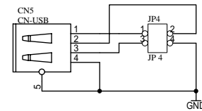
USB-IP
