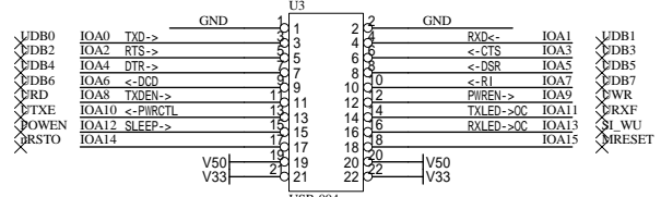
USB-004
