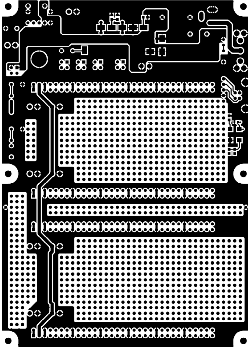
TOP LAYER
