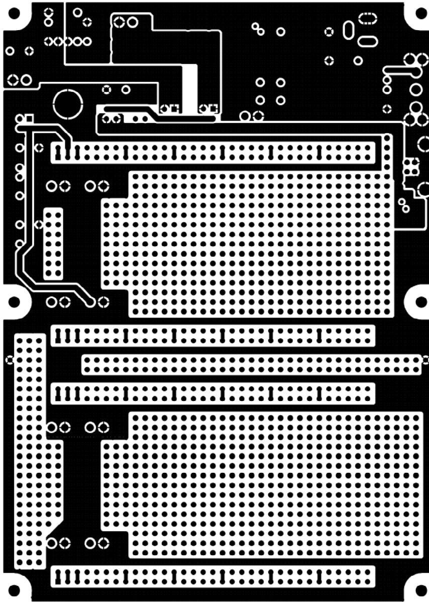
BOTTOM LAYER
