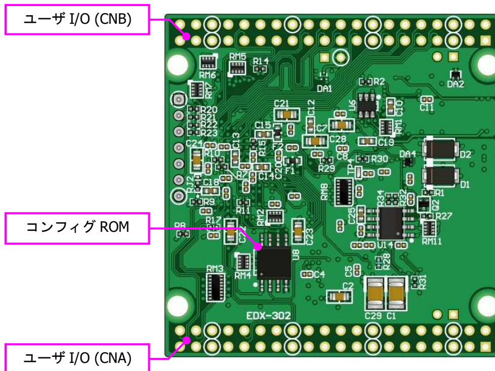
はんだ面
