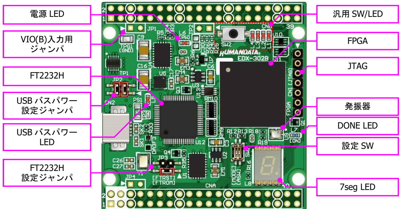
部品面
