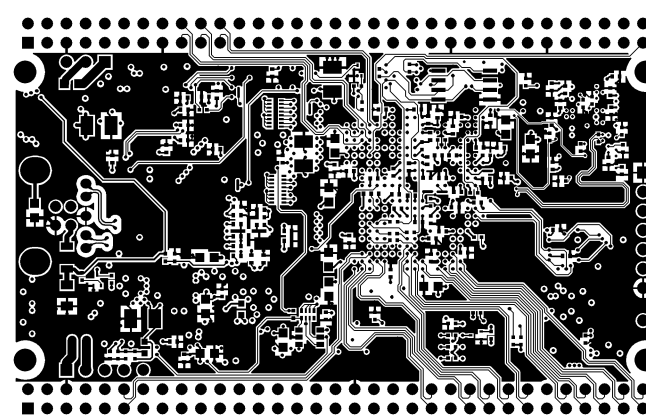
BOTTOM LAYER
