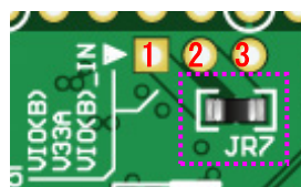
はんだ面
