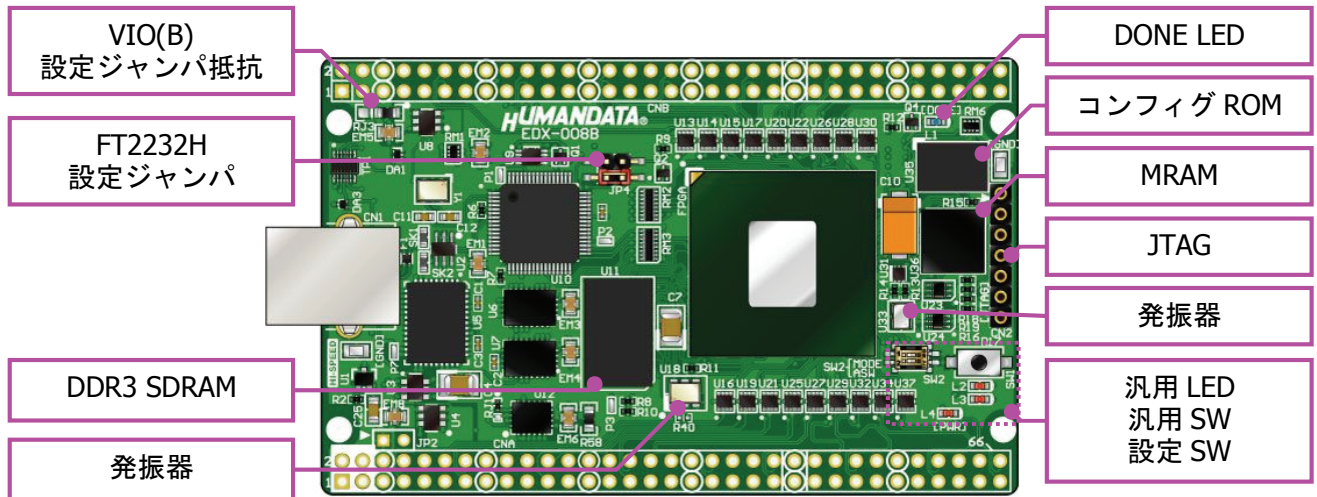
部品面
