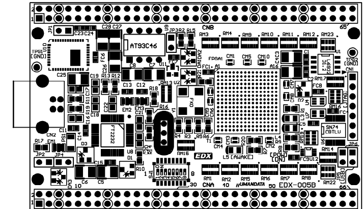
部品面
