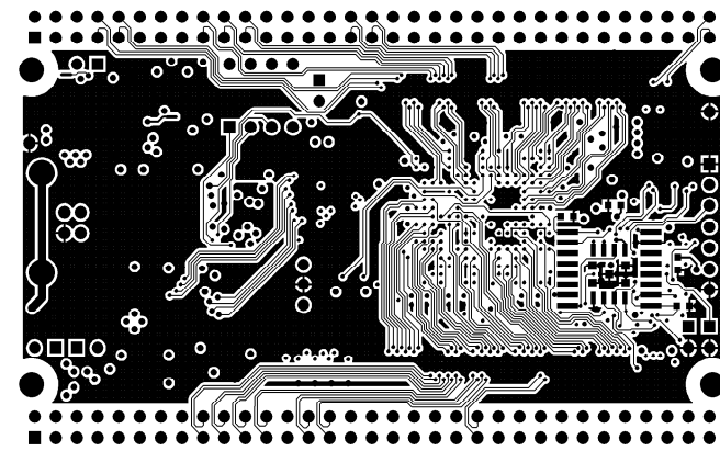
BOTTOM LAYER
