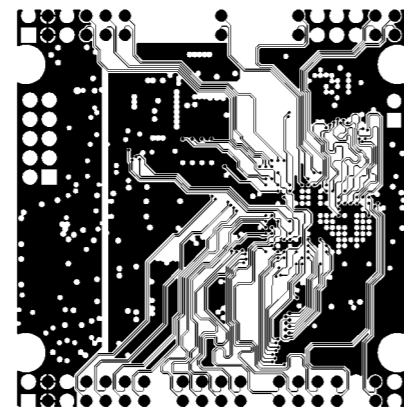
MID LAYER1
