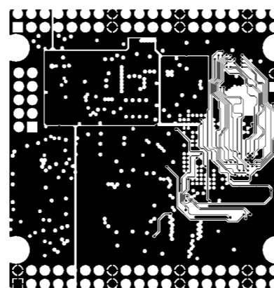
MID LAYER2
