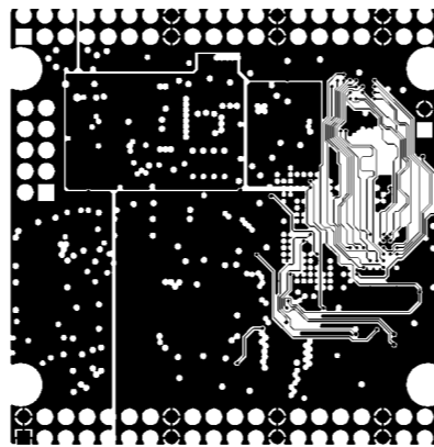
MID LAYER2
