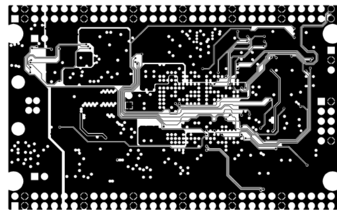
MID LAYER1
