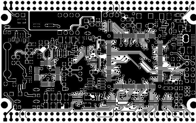
TOP LAYER
