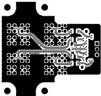
TOP LAYER
