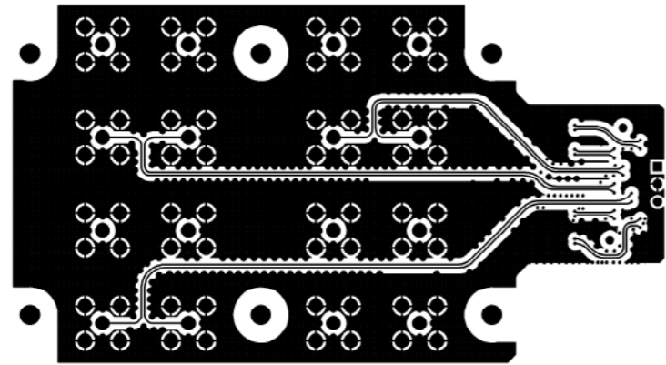
TOP LAYER
