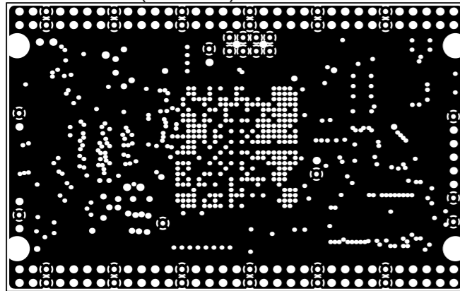
InternalPlane1 (Scale 1:1)
