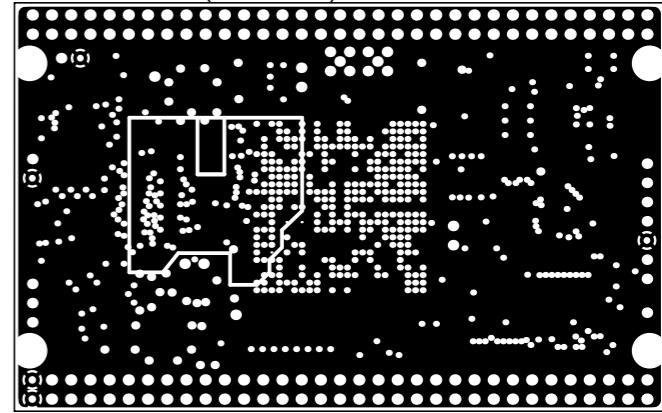
InternalPlane2 (Scale 1:1)
