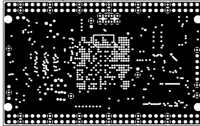
InternalPlane3 (Scale 1:1)
