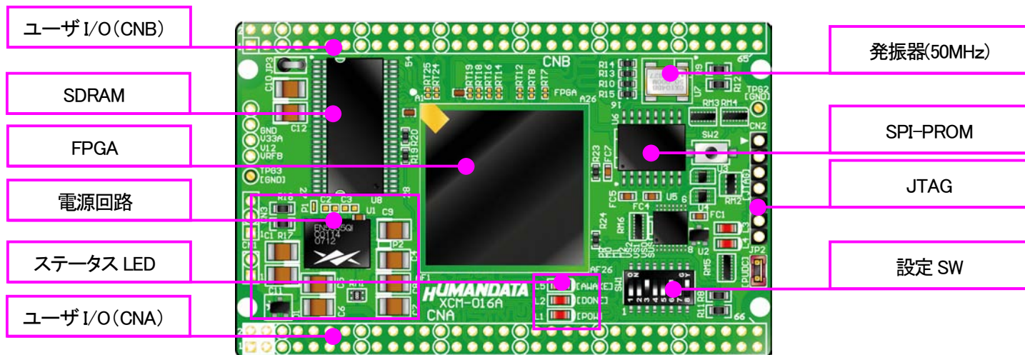
部品面
