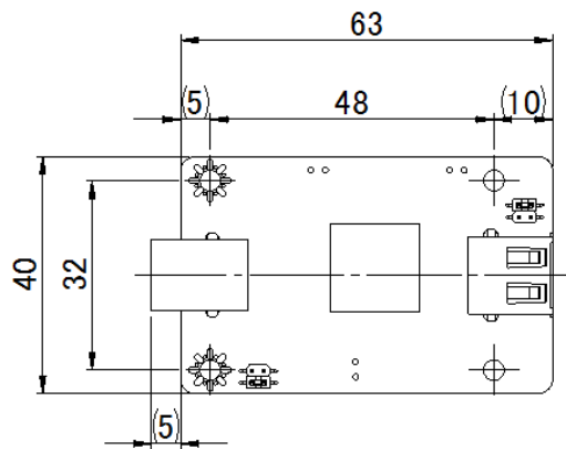
外形図 (mm)
