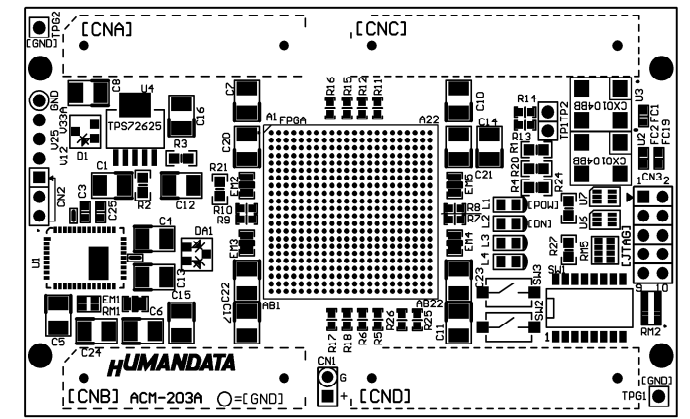
部品面
