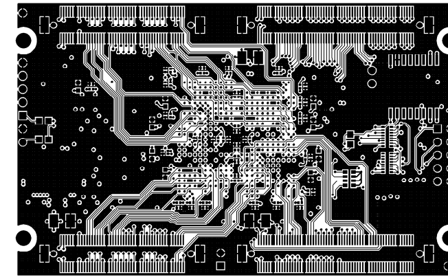
BOTTOM LAYER
