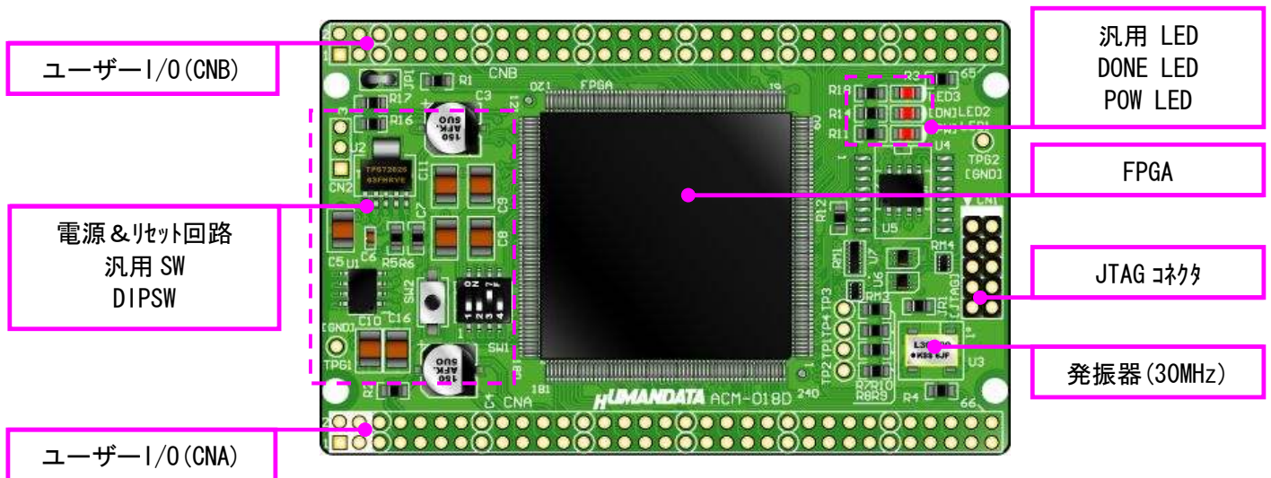
部品面
