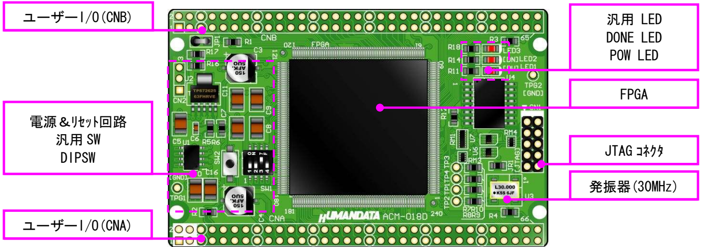
部品面
