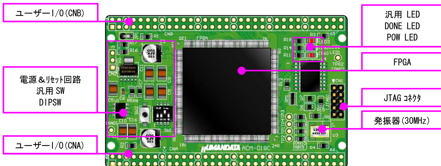
部品面
