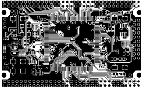
TOP LAYER
