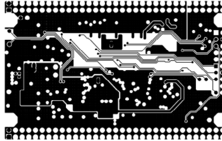
MID LAYER1
