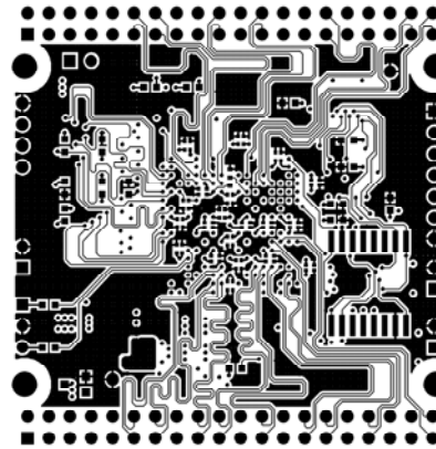
BOTTOM LAYER
