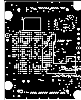
InternalPlane2 (Scale 1:1)
