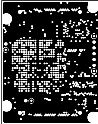
InternalPlane1 (Scale 1:1)
