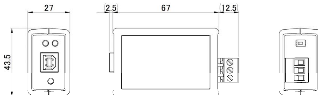
外形図 (mm)
