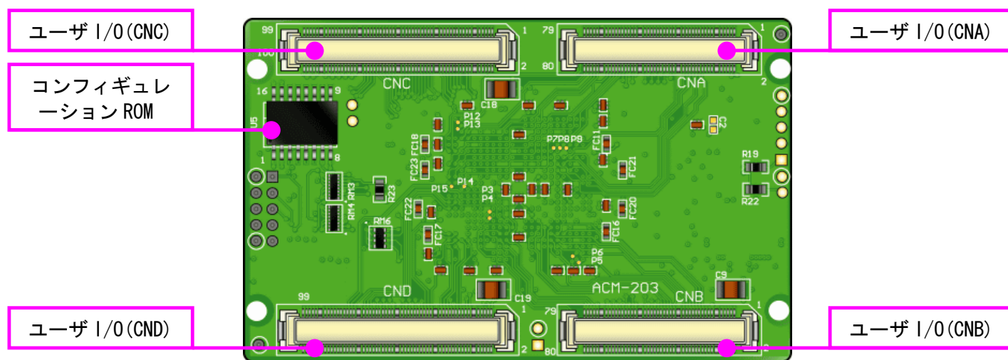
はんだ面
