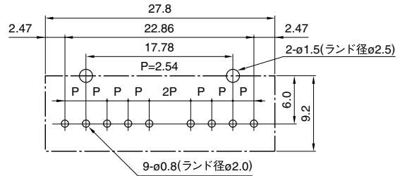
推奨基板取付け寸法
