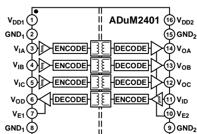
図 2. ADuM2401
