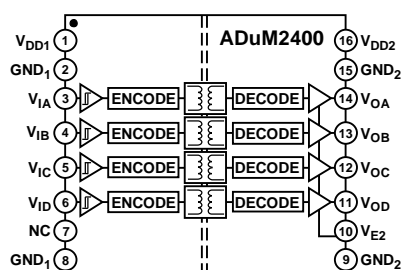
図 1. ADuM2400
