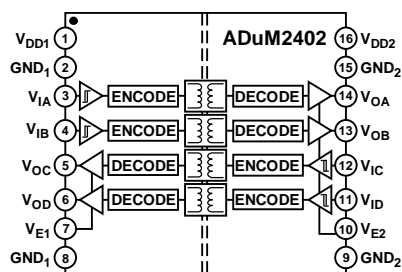
図 3. ADuM2402
