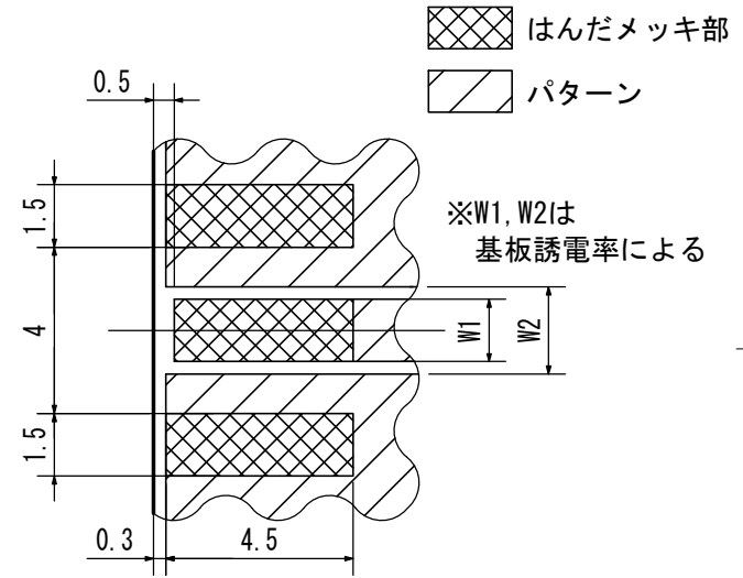
参考実装パターン (コプレナーの場合)
